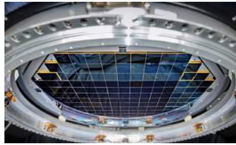
Câmera do telescópio LSST do Observatório Rubin terá 189 sensores individuais
